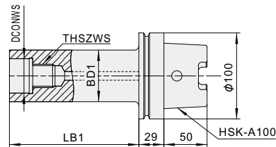
Fig.6 ボア(φ50,φ63)タイプ用アーバ Arbor for Bore(φ50,φ63) type
