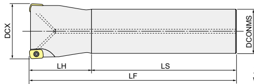
Fig.2 (アンダーカット形) Undercut type
