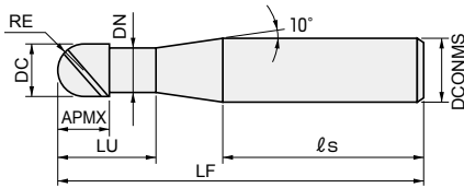
Aタイプ A type
