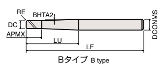
Bタイプ B type
