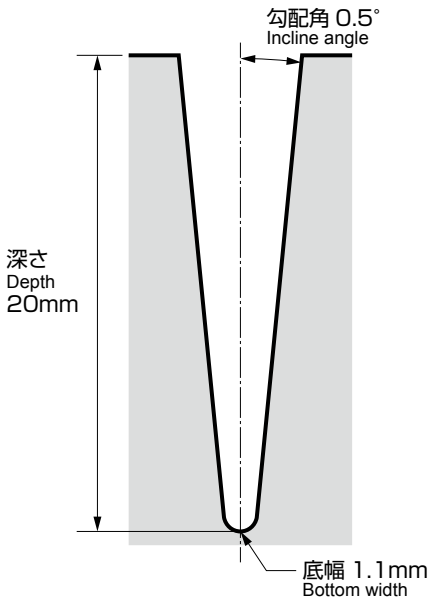
リブ溝形状 Rib groove profile
