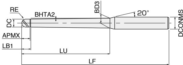
Aタイプ A type
