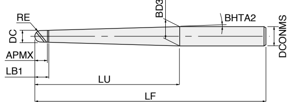
Bタイプ B type
