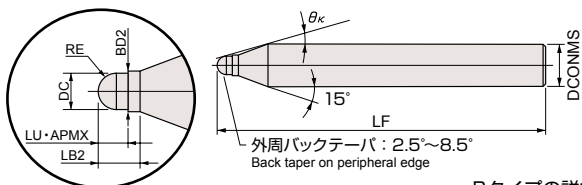
Bタイプ B type
