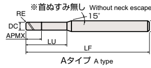
Aタイプ A type
